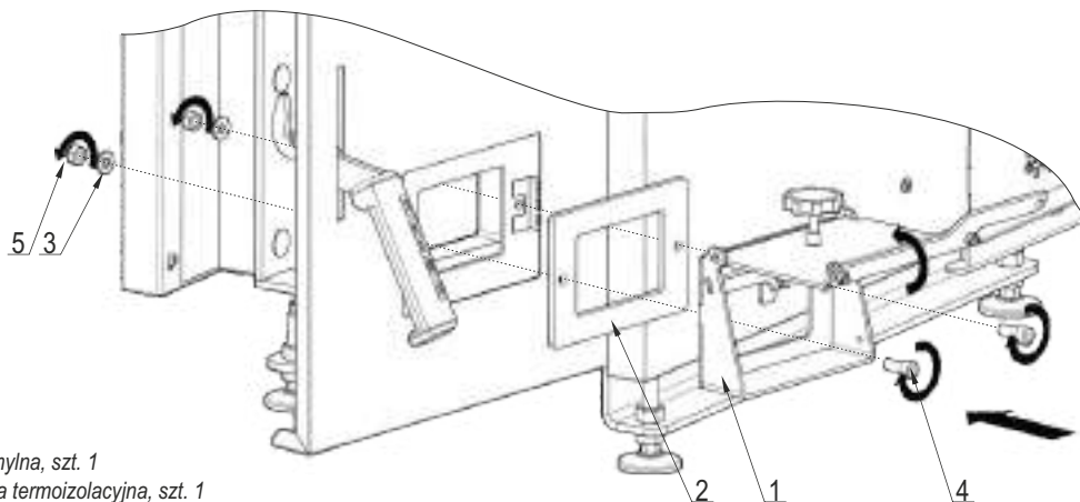
Rysunek 18. Instrukcja montażu klapy uchylnej.
